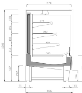
VBR12PDS
