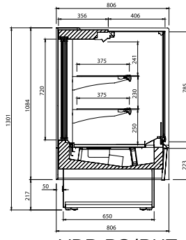
VBR PC/PHT
