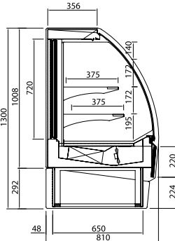
VBR HT
