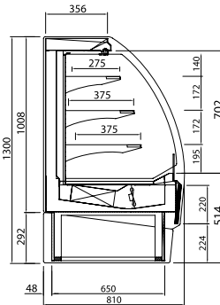
VBR SS
